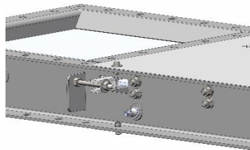
Stopfbuchse von außen nachstellbar
